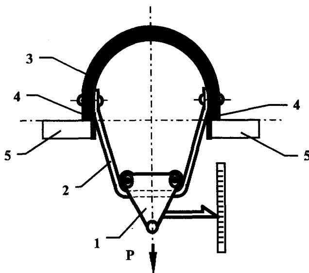
Рис. 2. Принципиальная схема устройства для проверки прочности подбородочного ремня:
